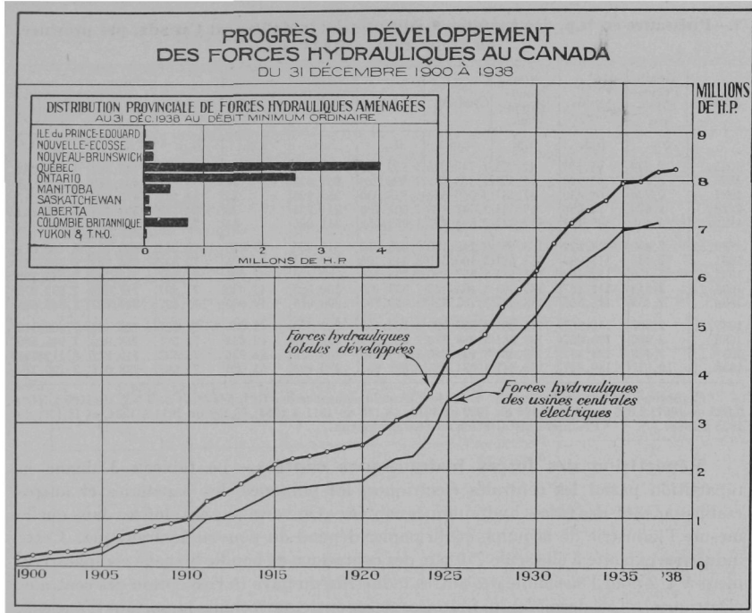
2.—Puissance en h.p. des turbines hydrauliques installées au Canada, par province, au 31 décembre 1900-38.
